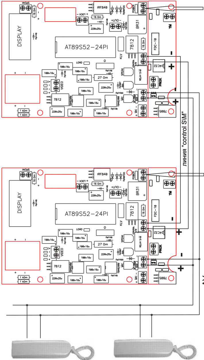
СХЕМА MASTER / SLAVE
